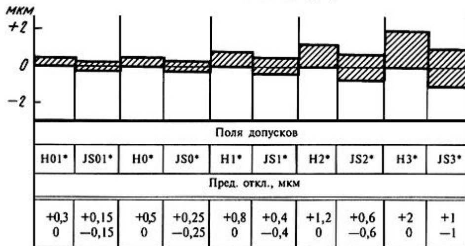
Поля допусков отверстий при номинальных размерах менее 1 мм. Предельные отклонения Квалитеты от 01 до 3
