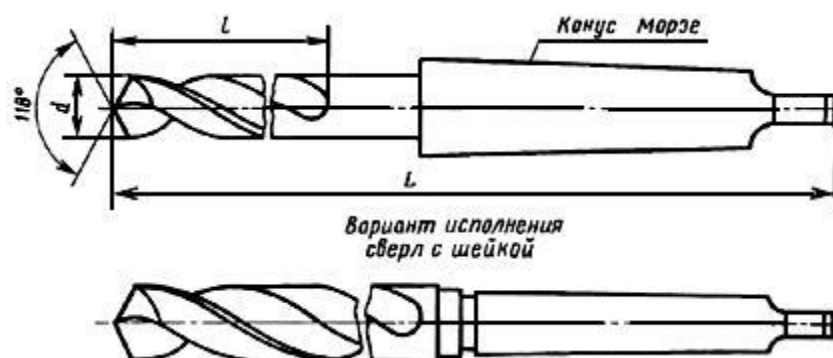
Чертеж. Основные размеры сверл
